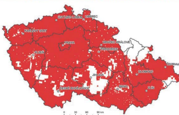
Oblasti ČR s překročenými imisními limity pro ochranu lidského zdraví (se zahrnutím přízemního ozonu), 2018
